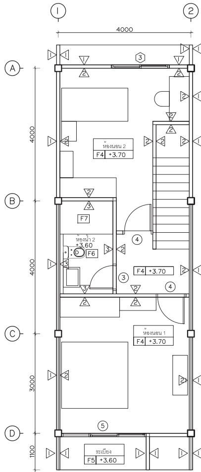
แปลนพื้นที่ 2 SCALE 1:75
