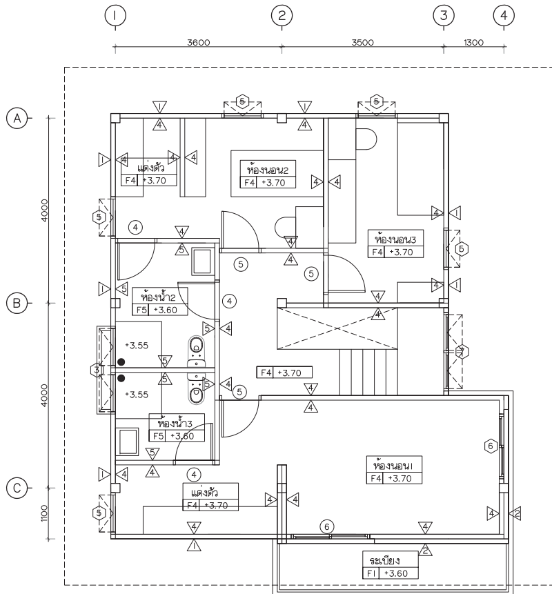
แปลนพื้นที่ 2 SCALE 1:75
