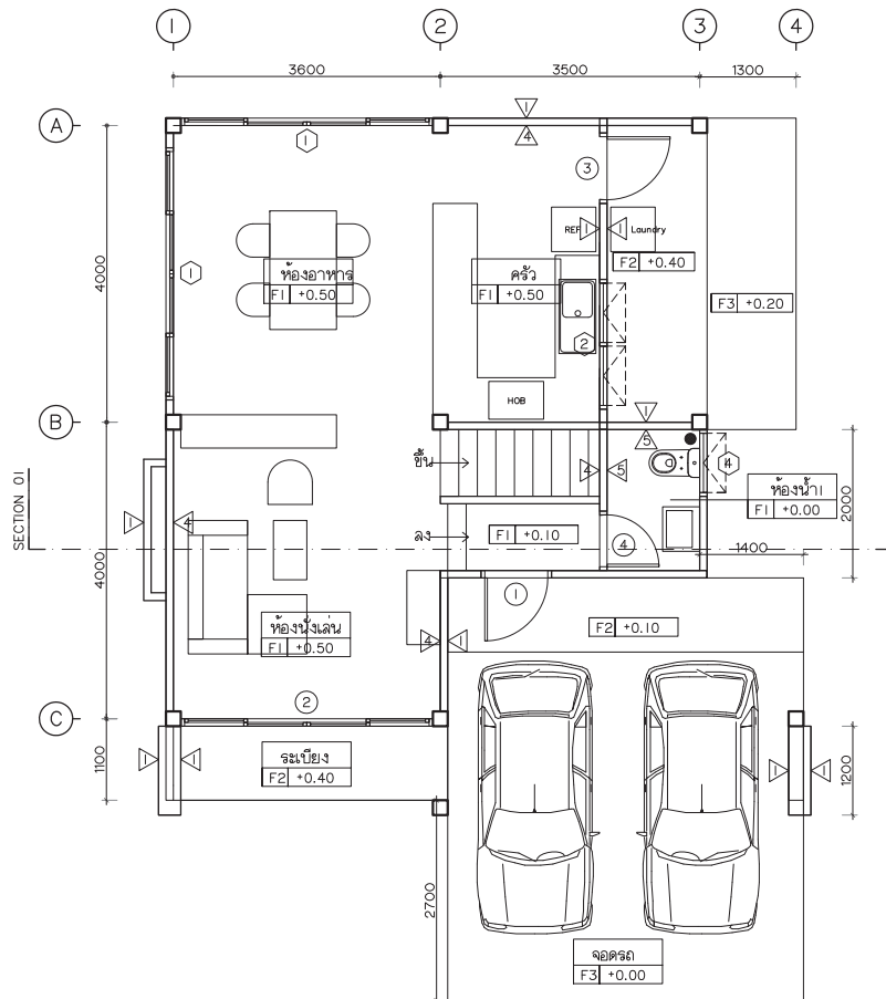
แปลนพื้นที่ 1 SCALE 1:75
